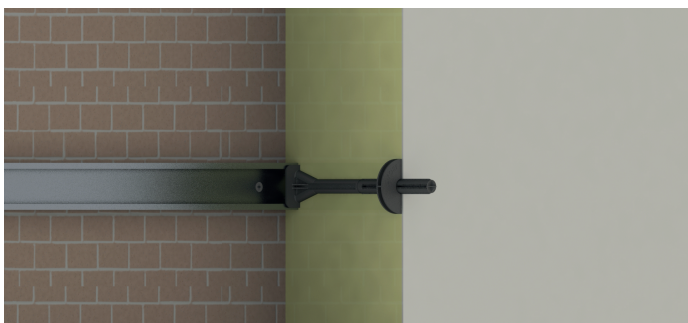
4. Positionner la membrane pare-vapeur Easyvap
