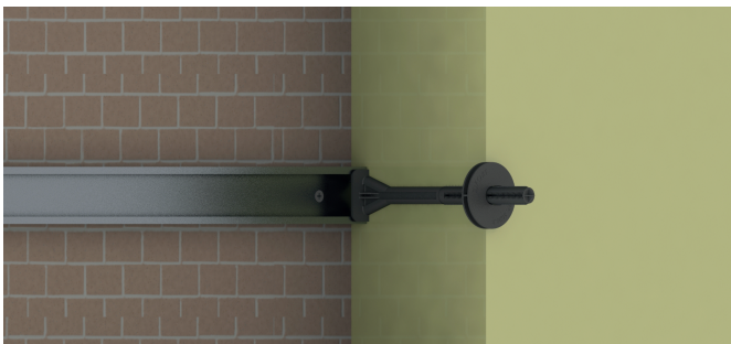
3. Fixer le contre-joint
