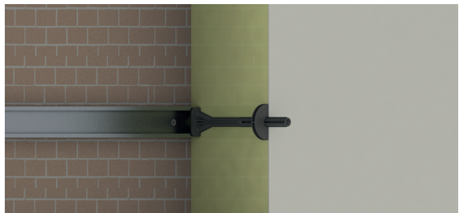
4. Positionner la membrane pare-vapeur Easyvap
